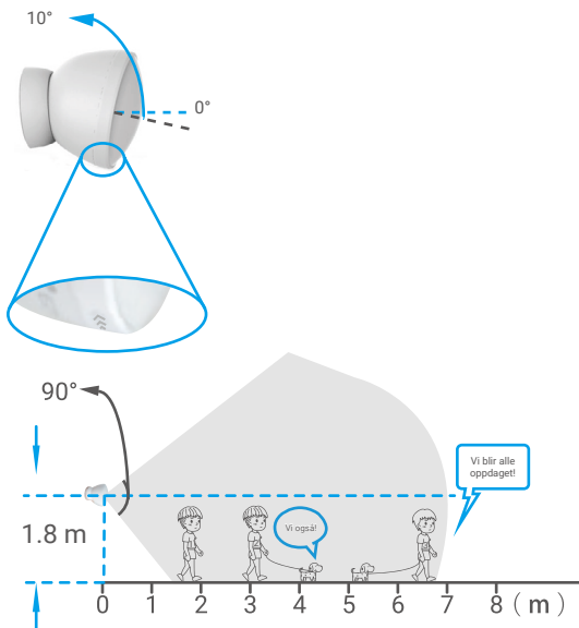
Fig. 1 Deteksjonsområdet sett fra siden
