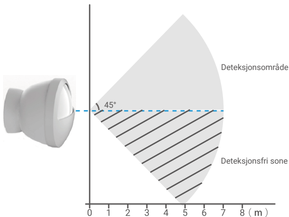
Fig. 2 Visning av deteksjonsområdet sett ovenfra
