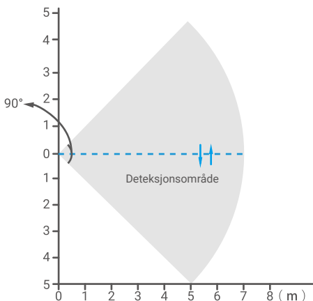
Fig. 2 Visning av deteksjonsområdet sett ovenfra
