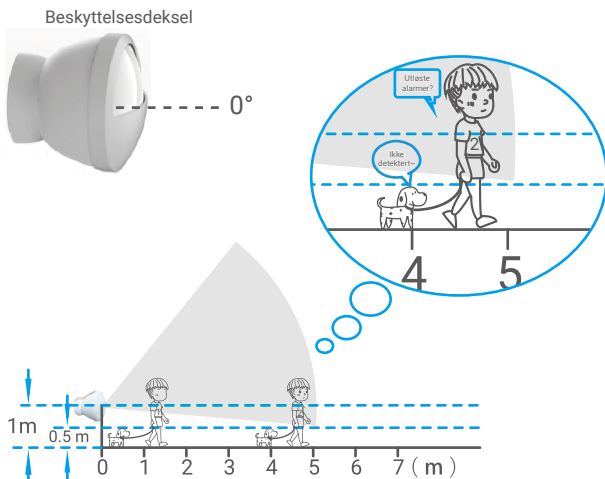
Fig. 1 Deteksjonsområdet sett fra siden
